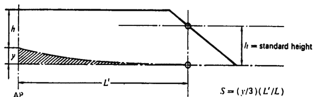
Σχήμα 38.3 Έκπτωση σιμότητας S για περίσσεια ύψους
